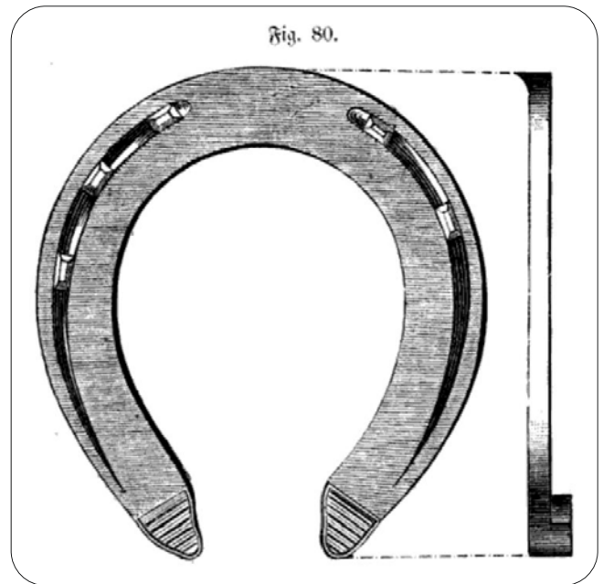
Abb. 4: Bodenfläche eines bestellten Hufeisens mit Sohlenabdachung (Görgch & Bauer 1876, p. 117) / Bottom surface of a horseshoe with studs and a concave section along the inner edge (Görgch & Bauer 1876, p. 117)
